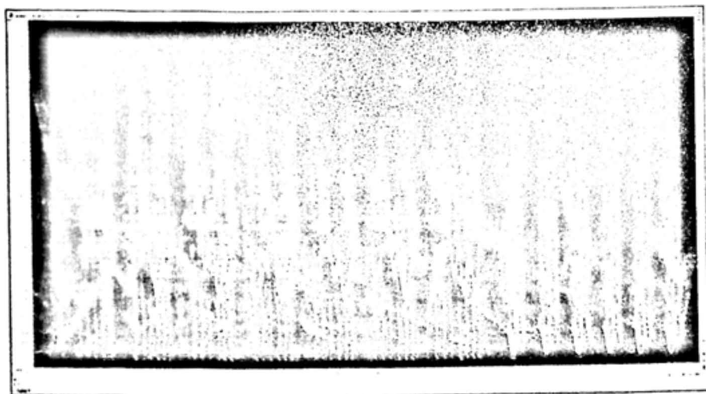
图47 一首座头鲸（bowhead whale）歌曲的声谱图。鲸鱼对这首歌有怎样的感受？原声带专辑《旅行者》中除了贝多芬、巴赫和查克·贝里之外，也录了一首鲸鱼歌，但我们只能希望这头鲸鱼真的唱得不错
