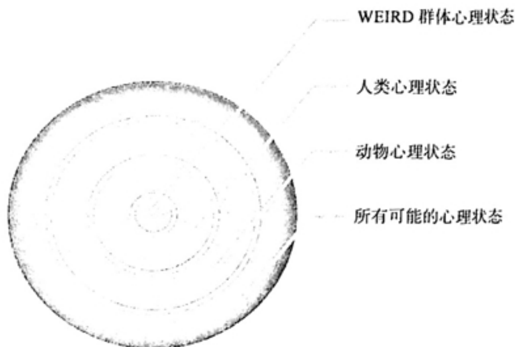
图 48 意识的频谱
