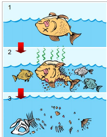
事实：鱼死后，浮在水面上，被吃掉，剩下的遗骸会分解。
