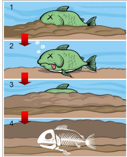
故事：鱼死后，沉入水底，逐渐被沉积物掩盖，石化。
