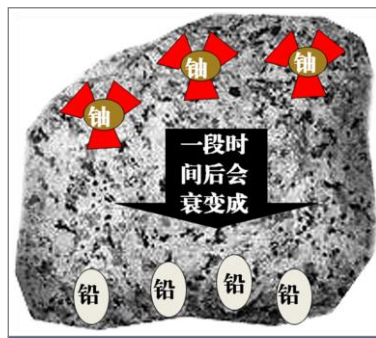
铀衰变为铅。
