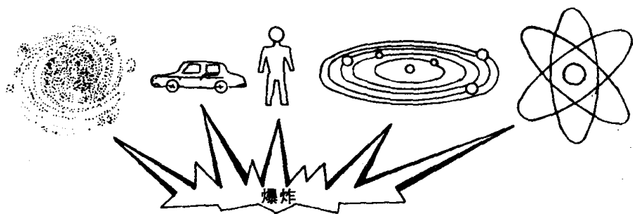
图6 从宇宙的混沌状态中如何生出了有序状态，这是个谜。现今的有序结构和复杂的活动不知是怎样从大爆炸杂乱无章的骚动中产生出来的。显然这违反了热力学第二定律。因为热力学第二定律说，随着时间的流逝，有序程度会降低而不是升高。解决这一难题可能得求助于引力的特异性质。
