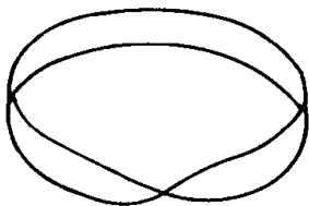
图 10 著名的莫比乌斯带。把一条带子扭转一下，使其两端连在一起，作成环。仔细观察就会发现，这带子现在只有一个面，也只有一条边。
