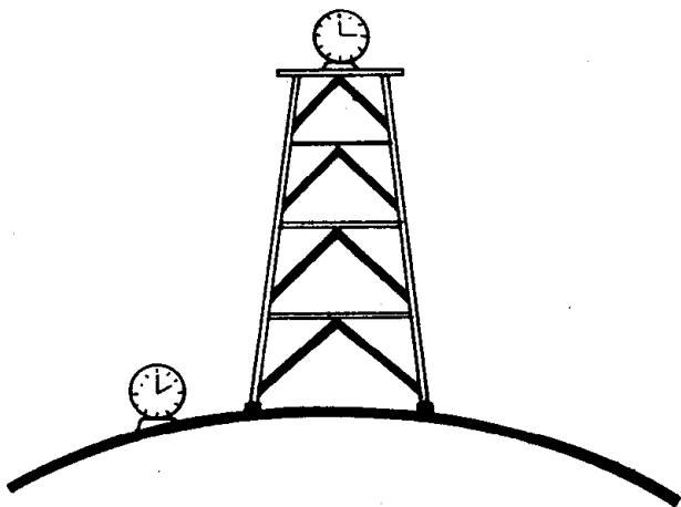
图 20 引力使时间减慢，这在地球上也可以用实验证明。相对于塔脚下的钟而言，塔顶上的钟走时快。
