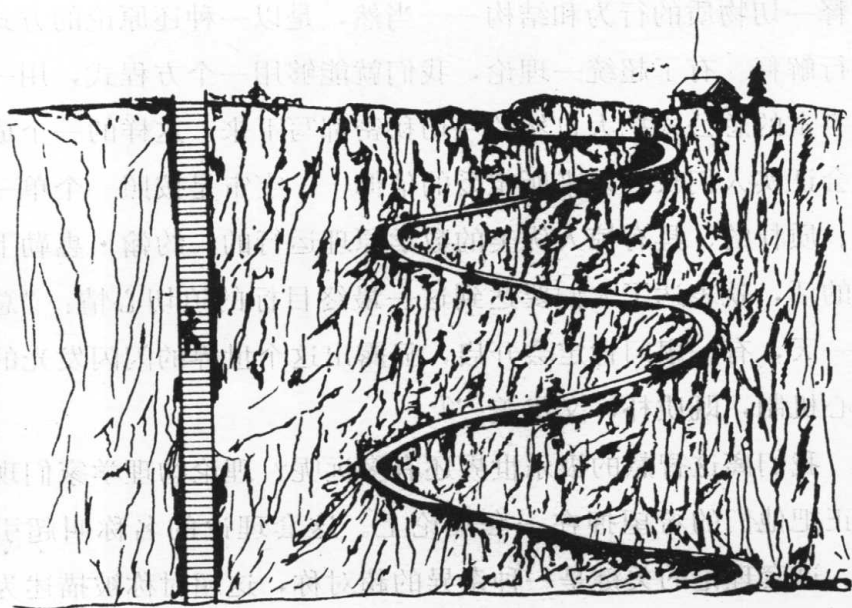
图 24 攀登断崖可以用来说明“规范对称”这一抽象的概念。不管是走那条直而短然而却是艰难的路，还是走那条长而易走的之字形路，攀上崖顶所需的全部能量是相同的。这反映的就是引力场深刻而有力的对称。大自然其他的力场与此相似而更为复杂的对称，最近在统一场理论的数学表达中得到了利用。
