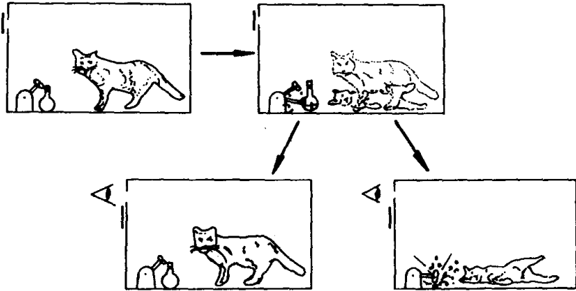
图 17 薛定谔猫的悲惨故事。一个量子过程可以 50 : 50 的概率使杀猫剂释放出来。量子论认为，整个系统必得进入幽灵般的混合状态，在进行观察之前，猫就是处于这种死-活的混合状态。一旦进行了观察，就会发现那猫不是活的就是死的。这种想象实验突出了量子论中观察行为的不可思议的含义。
