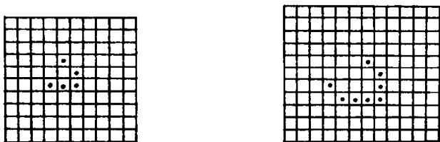
图 26 5 个小点简单地排列成“滑翔机”。这滑翔机有一个有趣的特征。它在板上作对角线运动，一直保持形状不变。由 8 个小点组成的图形叫“太空船”，但在运动时要喷射出“火花”。
