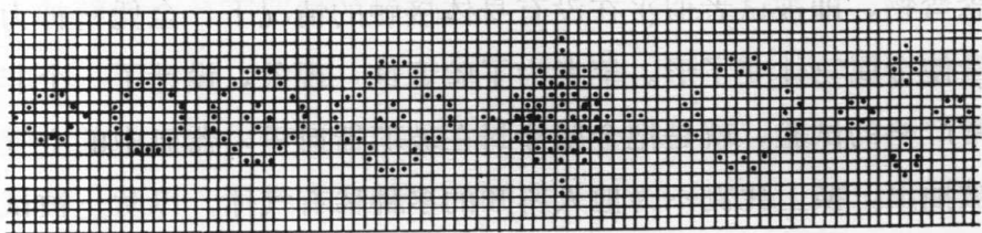
图 25 在约翰·康威的生命游戏里，有上面的一系列图形演变（有些中间步骤略去了）。这些图形恰巧像是一朵花的生命史。
