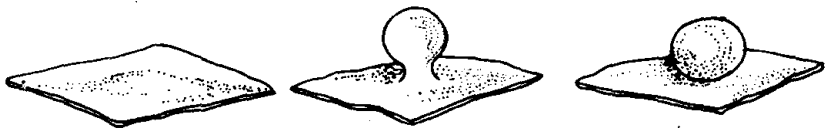
图5 爱因斯坦的广义相对论所提出的空间伸缩性，允许“子宇宙”（气球）从“亲宇宙”（胶皮）中生长并分离出来。这种拓扑变化是在近来的某些理论中被提出来的，但没有得到人们很好的理解。
