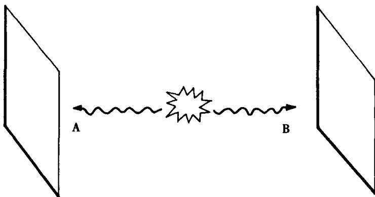
图 12 假如两个具有相关旋转和偏振的光子碰撞上平行的两块偏振材料，这两个光子就会显示出百分之百的合作：假如光子 A 被阻挡了，光子 B 也被阻挡。尽管 (1) 光子和起偏镜碰撞的实际结果是完全不可预测的，(2) 两个光子可能相距很远，但这种合作仍然发生。
