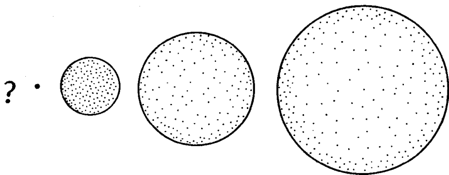
图 2 假如三维空间用一个二维的面来表示的话，那么，就可以有一个膨胀宇宙的模型，看上去很像是从无限小膨胀起来的气球。在这个模型里，空间是有限的，但也是无界的，在该空间中的一个观测者可以无障碍地漫游该空间。其中的小点代表星系（或星系团）。随着宇宙的膨胀，空间也拉长了，因而所有的小点都与其近邻的小点拉开了更大的距离。处在任何一个点上的观测者都会看到，其他的所有小点都在有条不紊地后退，而且他还会觉得他所在的小点是其他小点作四散运动的中心。
