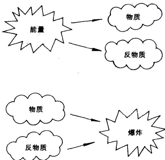
图4 在实验室中，可以用能量创造物质，但是，物质总是与等量的反物质一起出现的。当物质和反物质相遇时，就会发生爆炸，使双方湮灭。同时放出锁闭在物质中的能量。人们不知道，宇宙间的一切物质是怎么被创造出来，同时又没有掺上可以使其爆炸湮灭的反物质。
