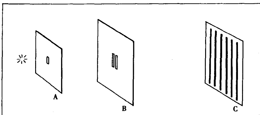
图 14 著名的杨氏双缝实验典型地揭示了光的奇妙的波-粒二象性（此实验也可用电子或其他粒子来做）。屏幕 A 上的小孔照亮了屏幕 B 上的两个狭缝。两个狭缝的影像显示在屏幕 C 上。显示出来的，并不是两道光，而是一系列明、暗条纹（即干涉条纹）。形成干涉条纹，是因为从两个狭缝发出的光波在某些位置上是同步到达屏幕 C 的，在另一些位置上则是不同步的。即使每一次只有一个光子通过实验装置，仍是照样形成同样的干涉条纹，尽管任何一个给定的光子只能经过屏幕 B 上两个裂孔中的一个，而且它也没有邻近的光子可用来为它量“步”。
