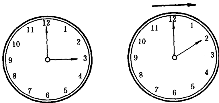
图 19 时间膨胀效应在对物理学家们来说已是司空见惯了。可以用高速运动的灵敏的原子钟或具有已知的衰变率的亚原子粒子显示出时间膨胀。运动的钟相对于不运动的钟而言，其走时要慢一些。这个现象就导致了著名的“双生子效应——一个宇航员高速航行若干年后返回地球，变得比他留在地球上的孪生兄弟年轻了。
